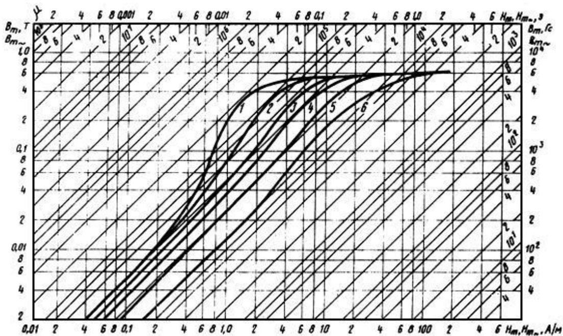
Кривые намагничивания сплава марки 80НХС толщиной 0,1 мм для частот:
