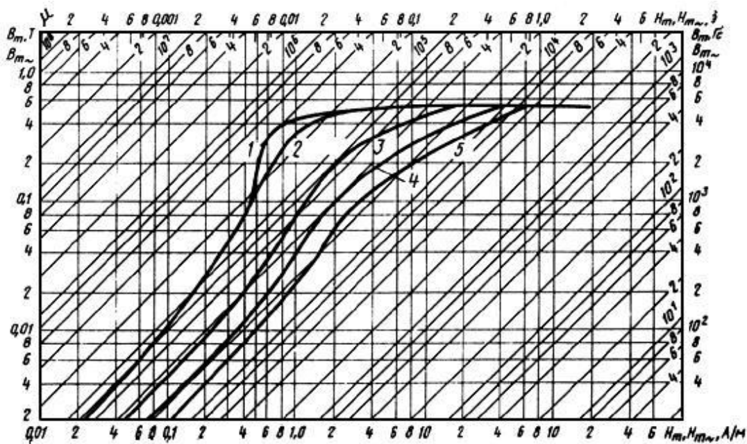
Кривые намагничивания сплава марки 81НМА толщиной 0,2 мм для частот:
