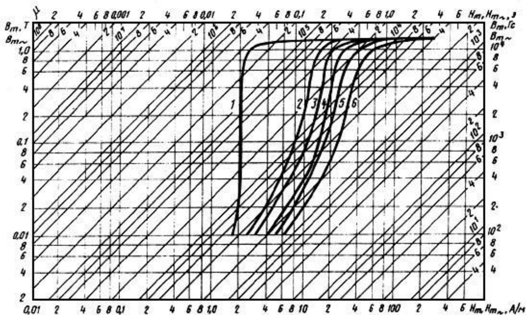
Кривые намагничивания сплава марки 40НКМП толщиной 0,05 мм для частот:
