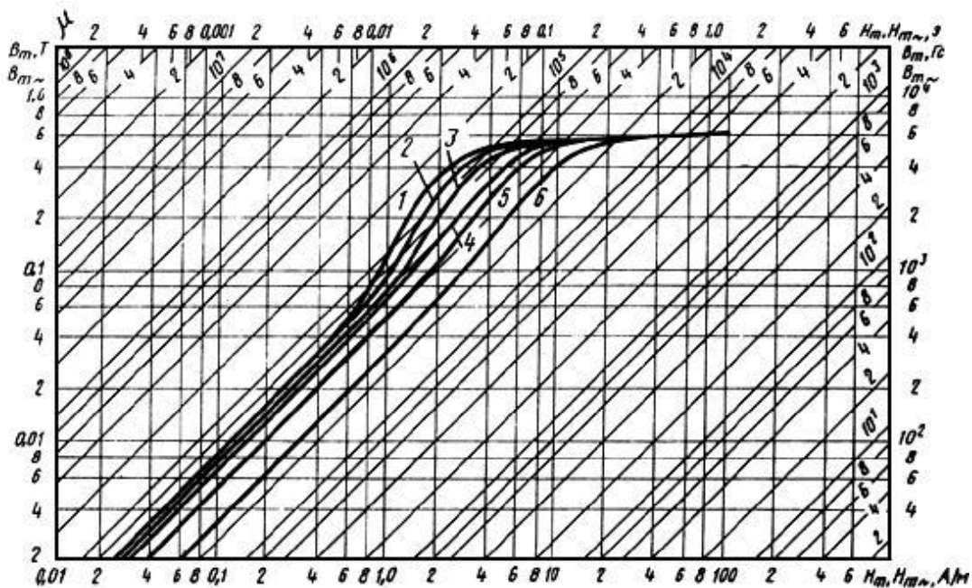
Кривые намагничивания сплава марки 83НФ толщиной 0,05 мм для частот:
