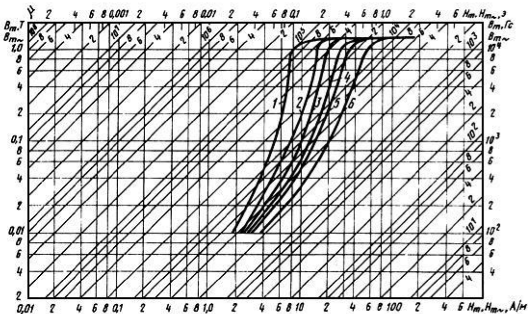
Кривые намагничивания сплава марки 34НКМП толщиной 0,05 мм для частот:
