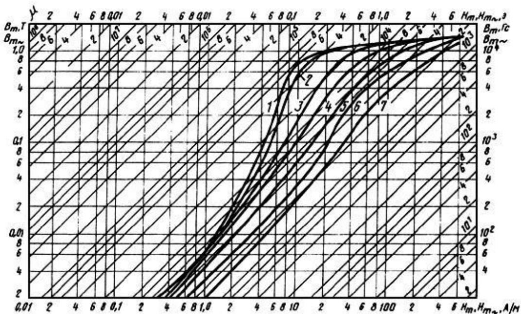
Кривые намагничивания сплава марки 50Н толщиной 0,2 мм для частот:
