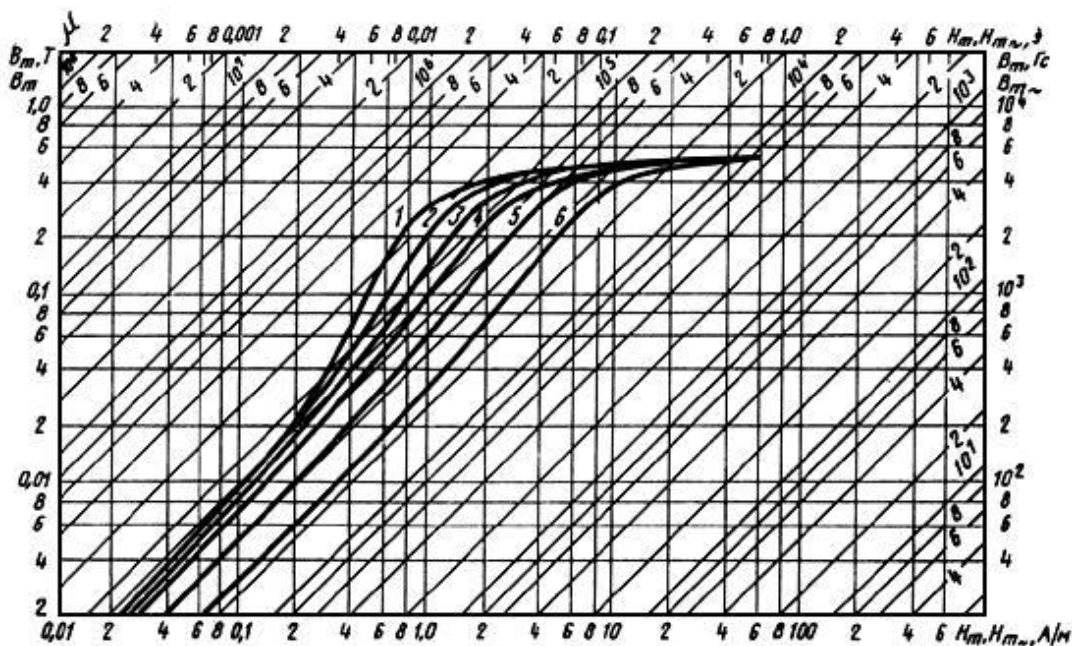
Кривые намагничивания сплава марки 81НМА толщиной 0,05 мм для частот:
