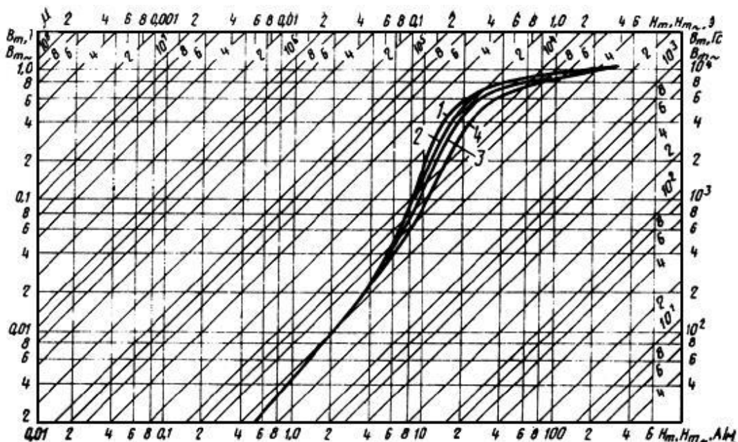
Кривые намагничивания сплава марки 50NХС толщиной 0,05 мм для частот:
