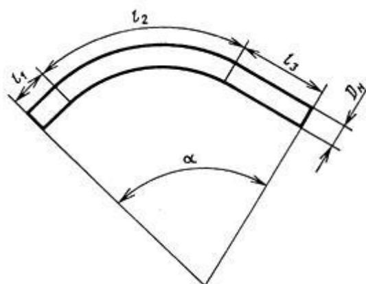
Отвод типа 1
